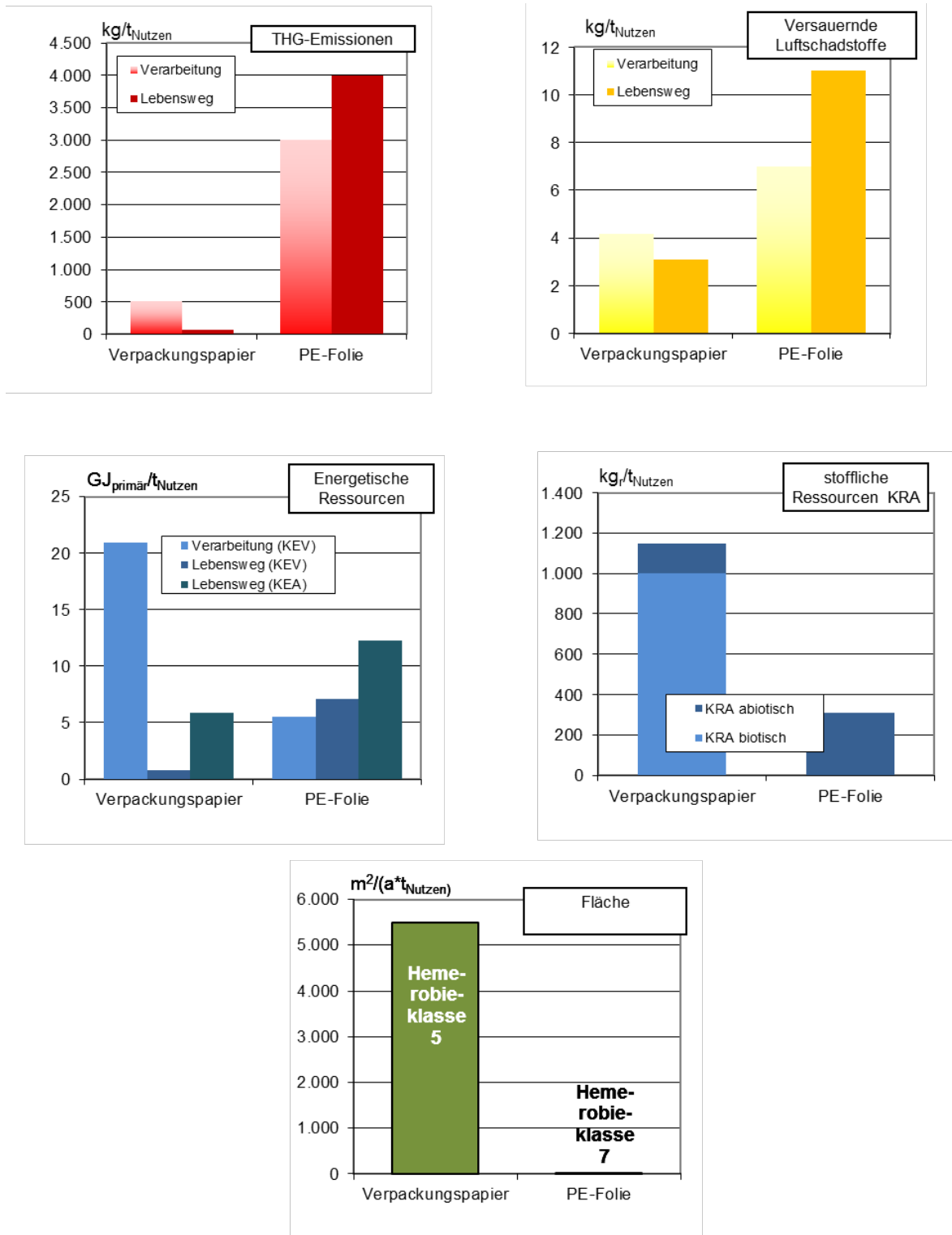
Abbildung 34: Ergebnisse der Indikatoren für das Substitutionspaar Verpackungspapier/PE-Folie
